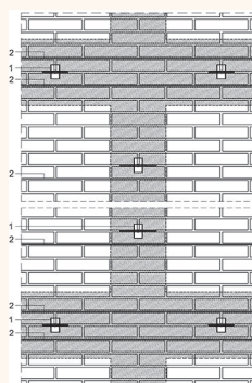
Imagen 5: Esquema del sistema G.H.A.S.
