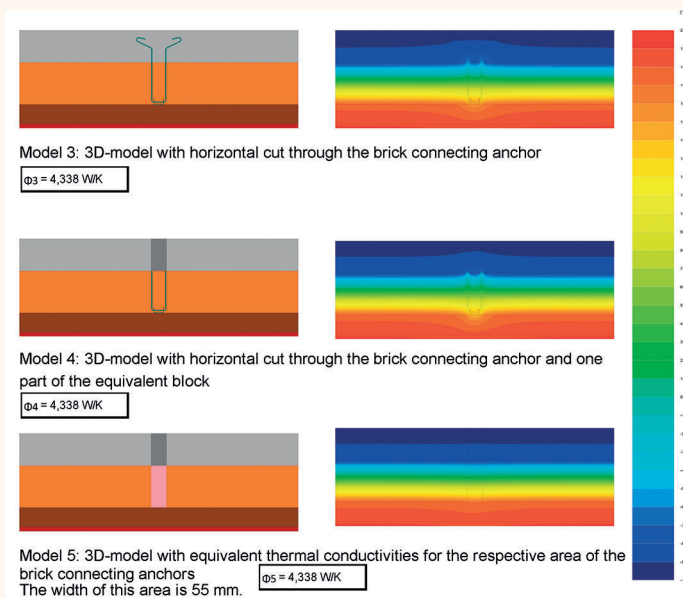
Imagen 6: Cálculo de la conductividad térmica equivalente de la cara exterior de ladrillo cara vista incluyendo los anclajes de retención GEOANC.
