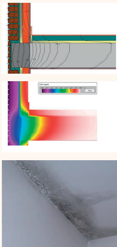
Imagen 3: Patologías ocasionadas por el puente térmico de un forjado de un sistema de fachada confinada
